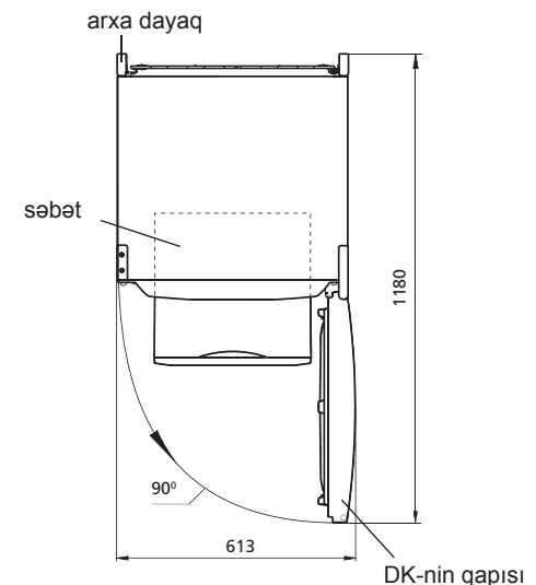
Şəkil 2 — Soyuducu (yuxarıdan görünüş)
